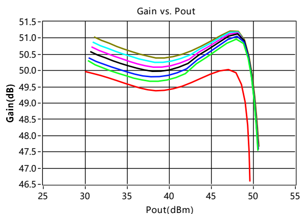
增益压缩
