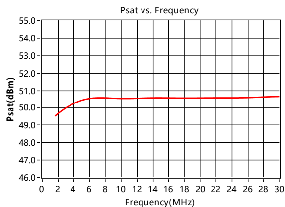
饱和功率
